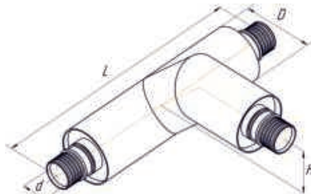
ГПИ пресс-тройник угловой равнопроходной
