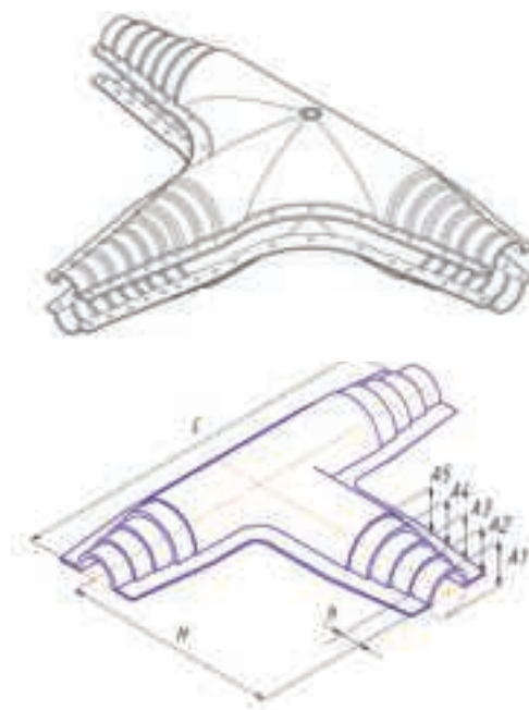
Кожух полимерный для изоляции пресс-тройника 225/160-225/160-225/160
