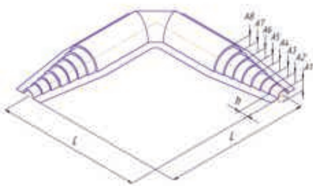
Кожух полимерный для изоляции пресс-отвода 160/63
