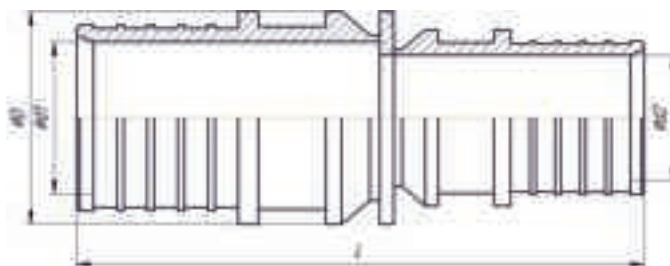
Пресс-муфта редукционная
