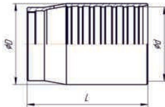
Гильза обжимная
