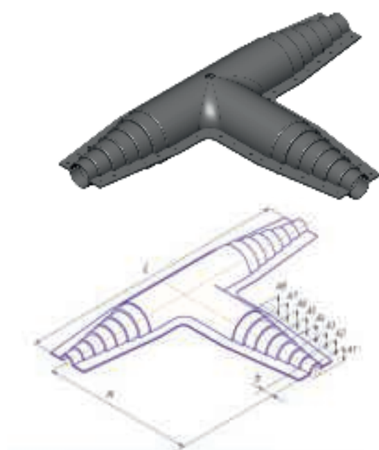
Кожух полимерный для изоляции пресс-тройника 160/63 - 160/63-160/63
