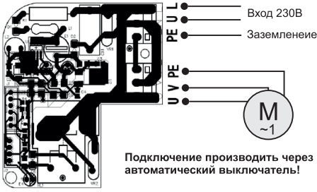
Схема подключения
